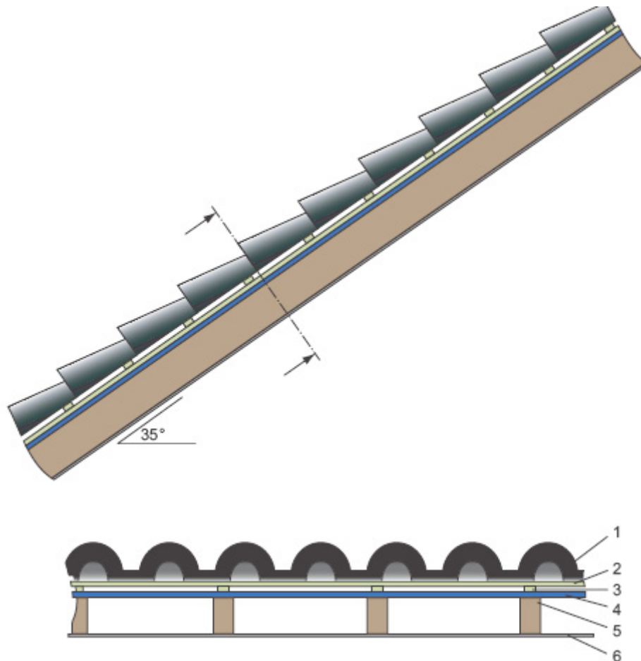
Afb. 1: Typische inbouwsituatie voor de composiet thermische isolatiedeken "Aluthermo Quattro" in een schuin dak, helling 35°, weergegeven in zijaanzicht en in doorsnede.
